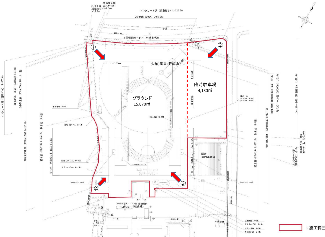
配置図
