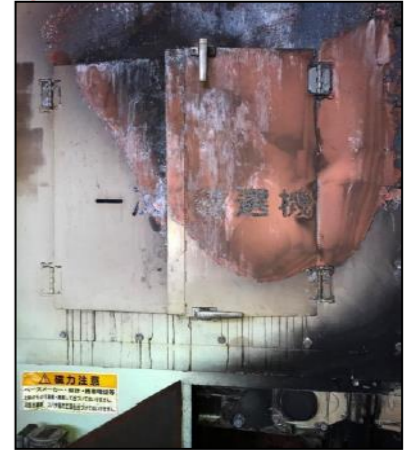
⑤一次磁選機（選別室6階側）
