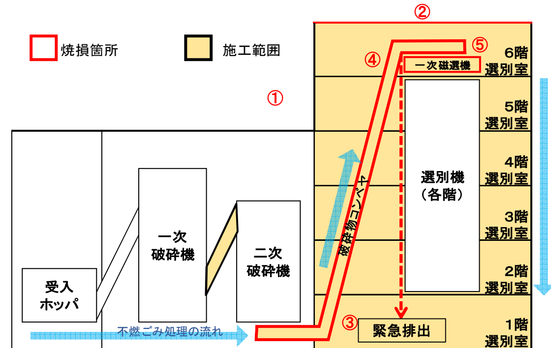
破碎選別処理施設フロー図（施工範囲）
