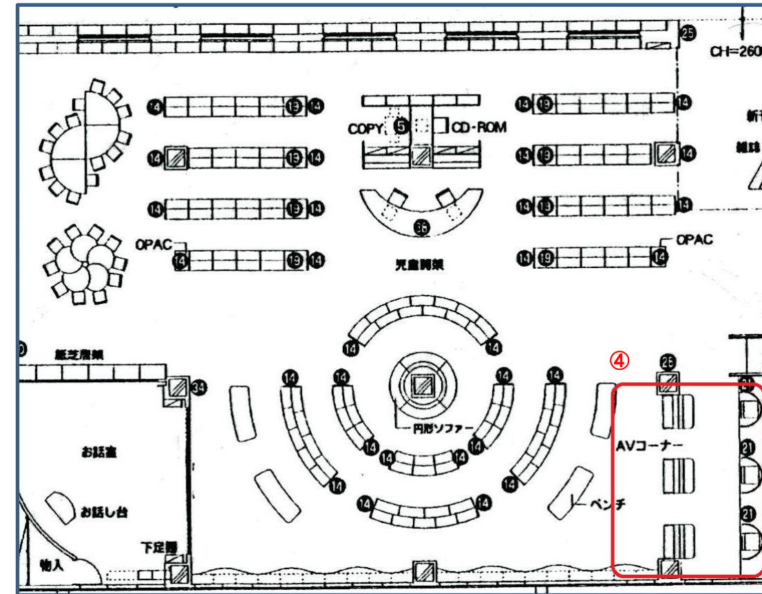
【7F 児童ライブラリー 図面】
